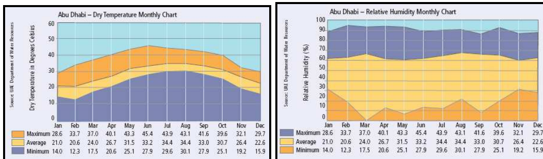
Εικ. 2.3, 2.4 – Ετήσια Διαγράμματα Θερμοκρασίας και Υγρασίας στα Η.Α.Ε.
